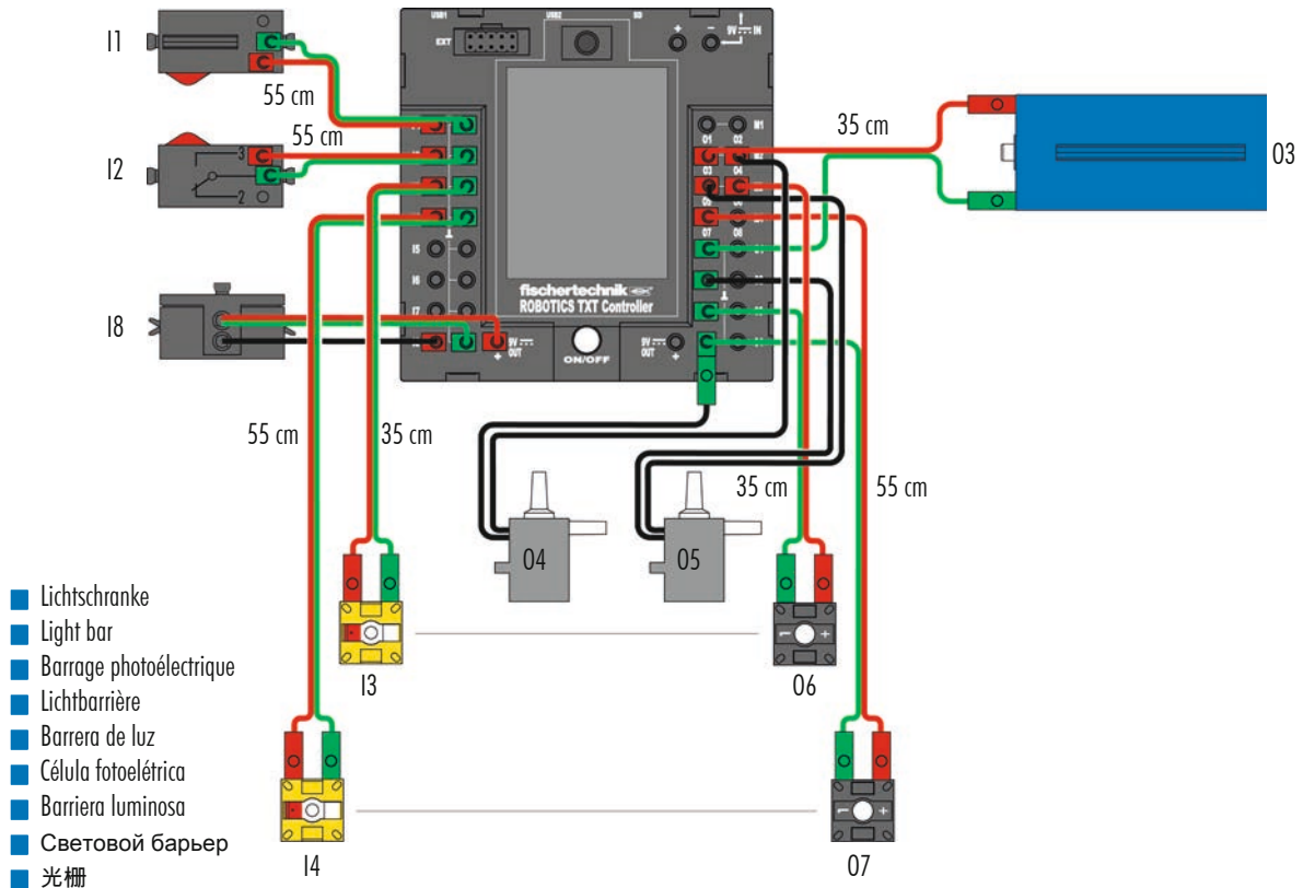
Schakelschema Diagrama de circuitos Plano eléctrico de ligação
